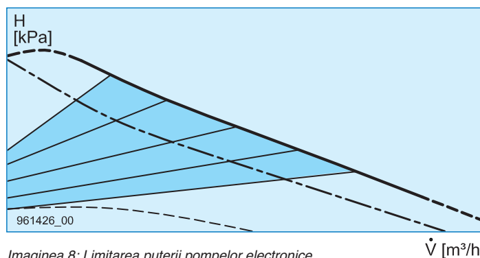
Imaginea 8: Limitarea puterii pompelor electronice ----- Limitarea puterii
